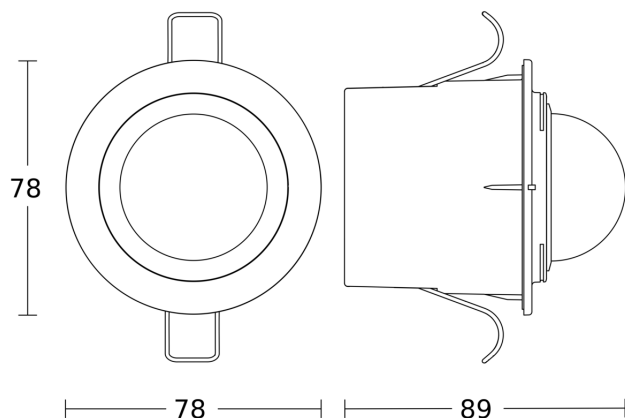
Dibujo acotado
